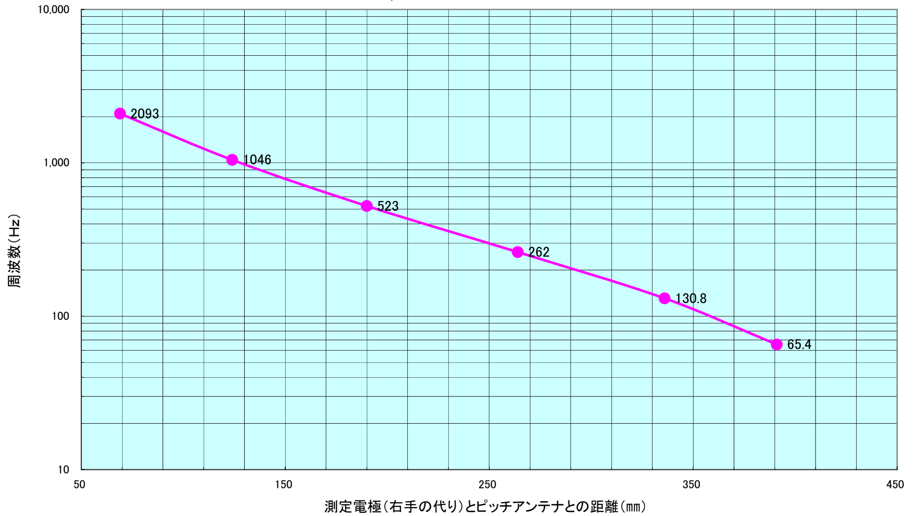
オクターブピッチ(C1-C6)特性 ゼロポイントを450mmにセット C1:65.4Hz、C2:130.8Hz ・ ・ C6:2093Hz
